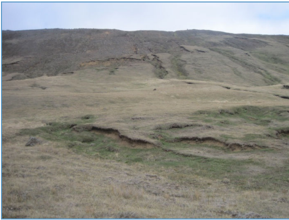
Mynd 1: Horft upp í rofabarðasvæði hjá bílagarðinum
