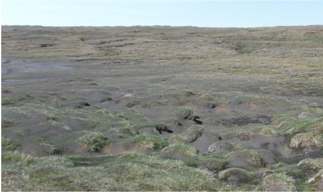
Mynd 14. Mikið áfok (4) frá suðri, úr lónstæði Háslóns
