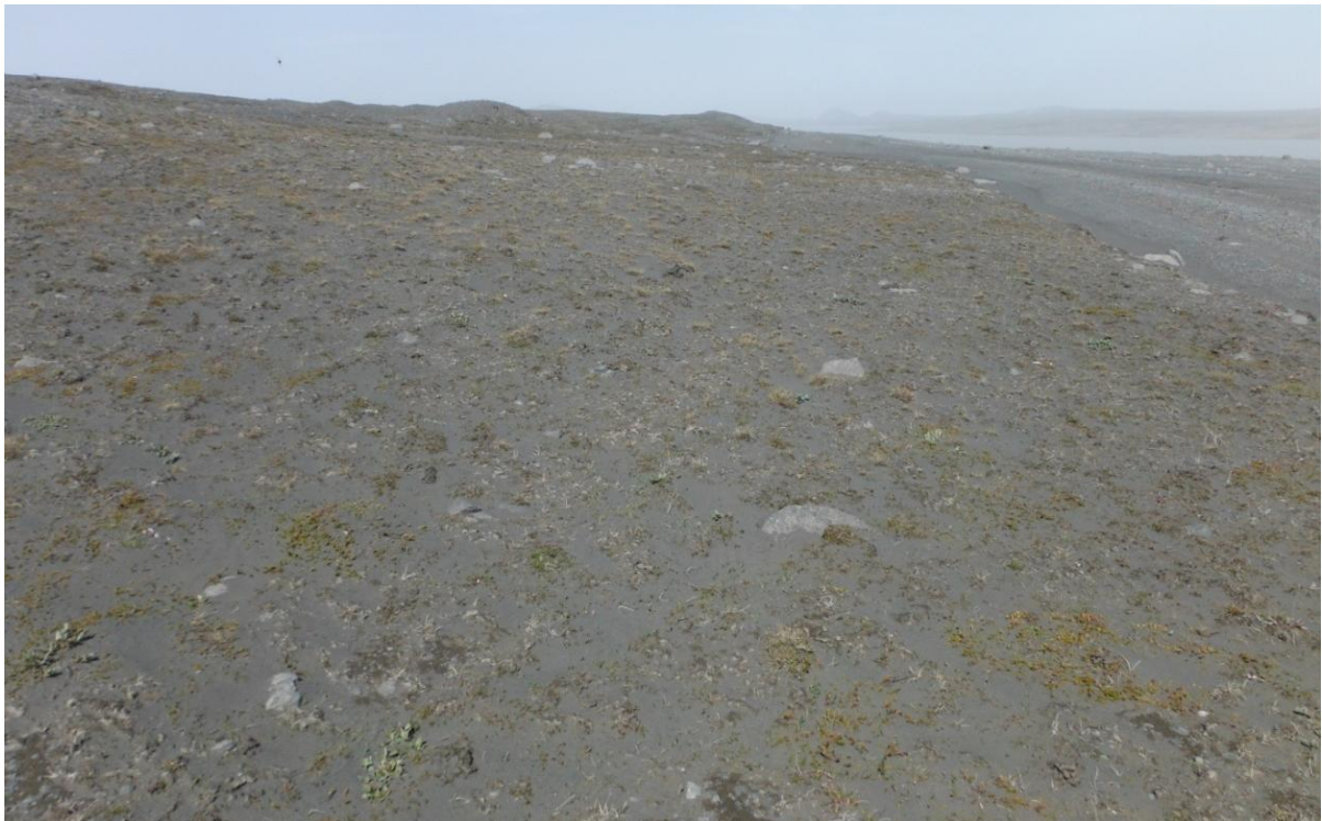
Mynd 16. Töluvert áfok (3) inn á gróið land við austurströnd Kringilsárrana
