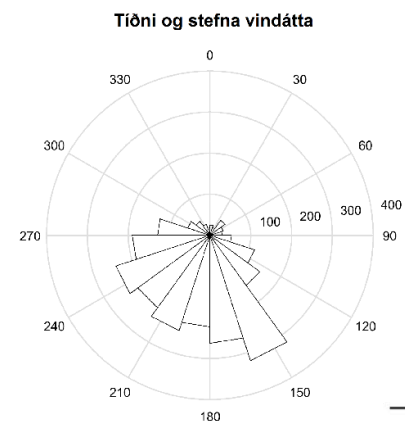
Mynd 18. Mælípúlssar (slög á tímaeiningu) og vindhraði ( m s^{-1} ) ásamt vindrósi fyrir tíðni og stefnu vindátta ( ^{\circ} ) á mælistöðvum A, B og C haustið 2015. Gröfin sýna 10 mínútna heildartalningar (slög sem mældust við <80\% loftraka, >4 m s^{-1} og >0^{\circ}C jarðvegshita) og 10 mínútna meðaltöl (vindhraði og vindátt). Eins og sjá má á mælistöðvum C þá mettast fokmælingarnar við 7999 mælípúlssa á tíu mínútum. Ath. að kvarðinn á tíðni vindátta er breytilegur milli vindrósa.
